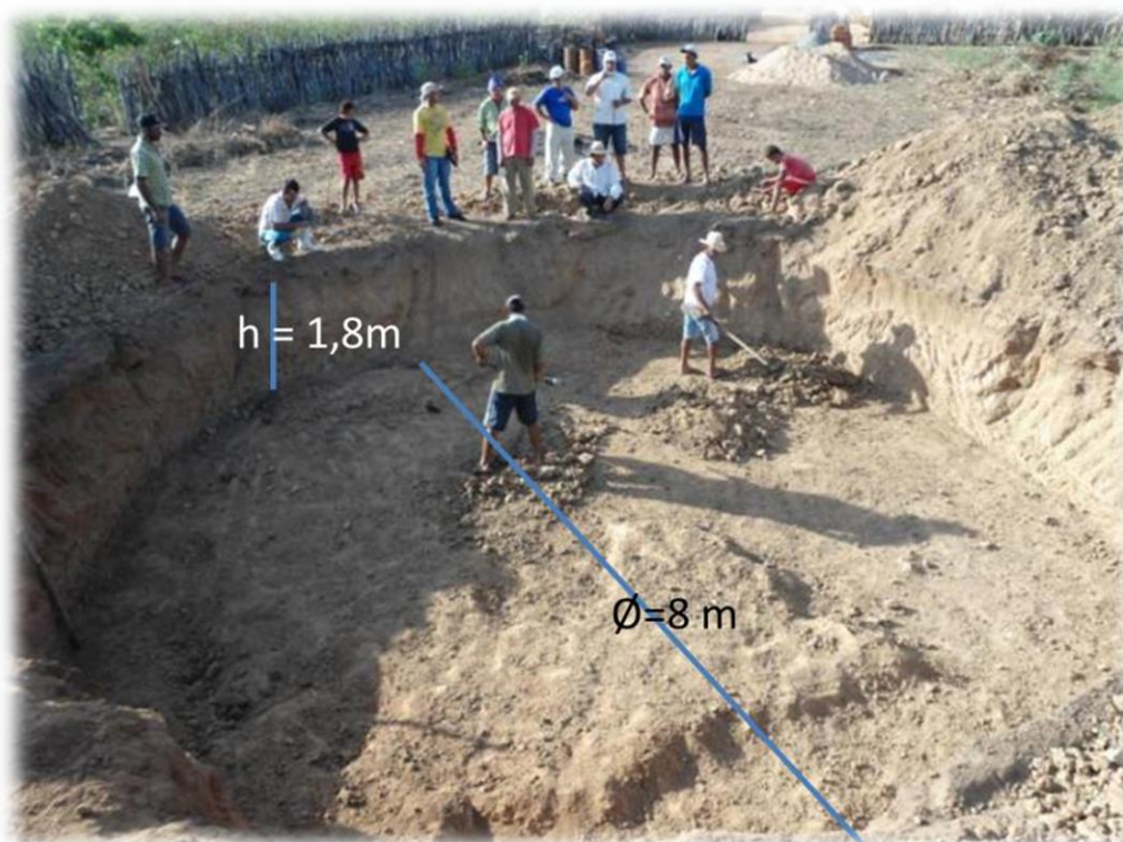
Figura 3: Escavação - acabamento manual do fundo da escavação
