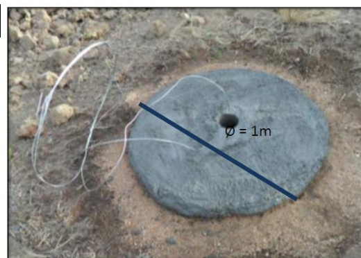
Figura 12. Confecção da bandeja de apoio ou coroa
