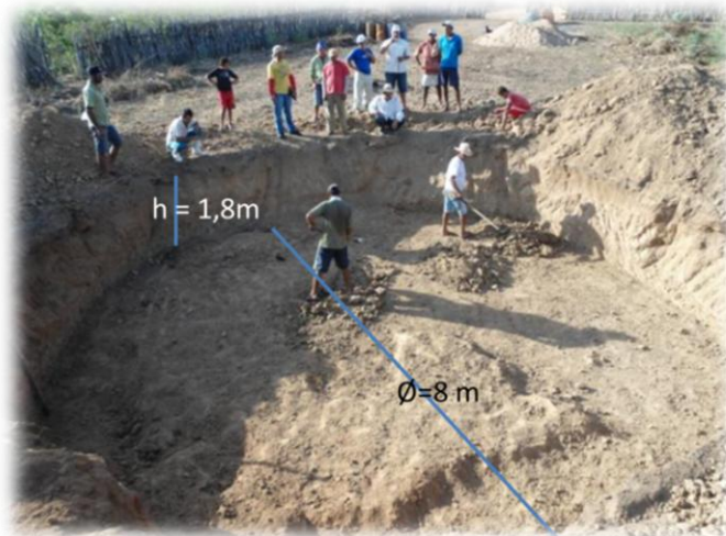
Figura 5. Acabamento manual do fundo da escavação
