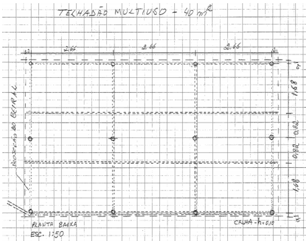
Figura 24 – Croquis da planta baixa do galpão
