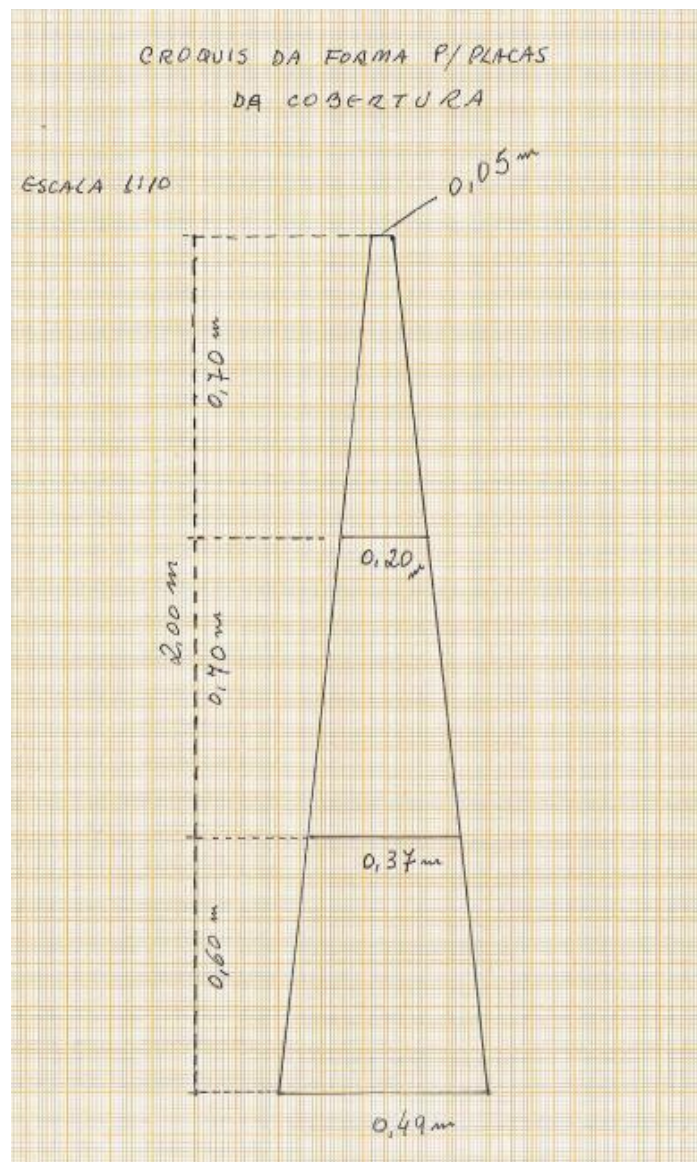
Figura 8 – Gabarito para confecção da forma das placas de cobertura
