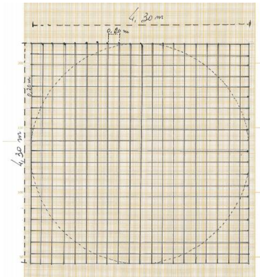
Figura 11 – Disposição dos vergalhões na armadura da laje de fundo da cisterna
