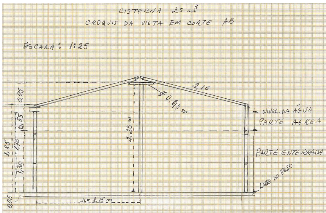
Figura 13 – Croquis da vista da cisterna em corte
