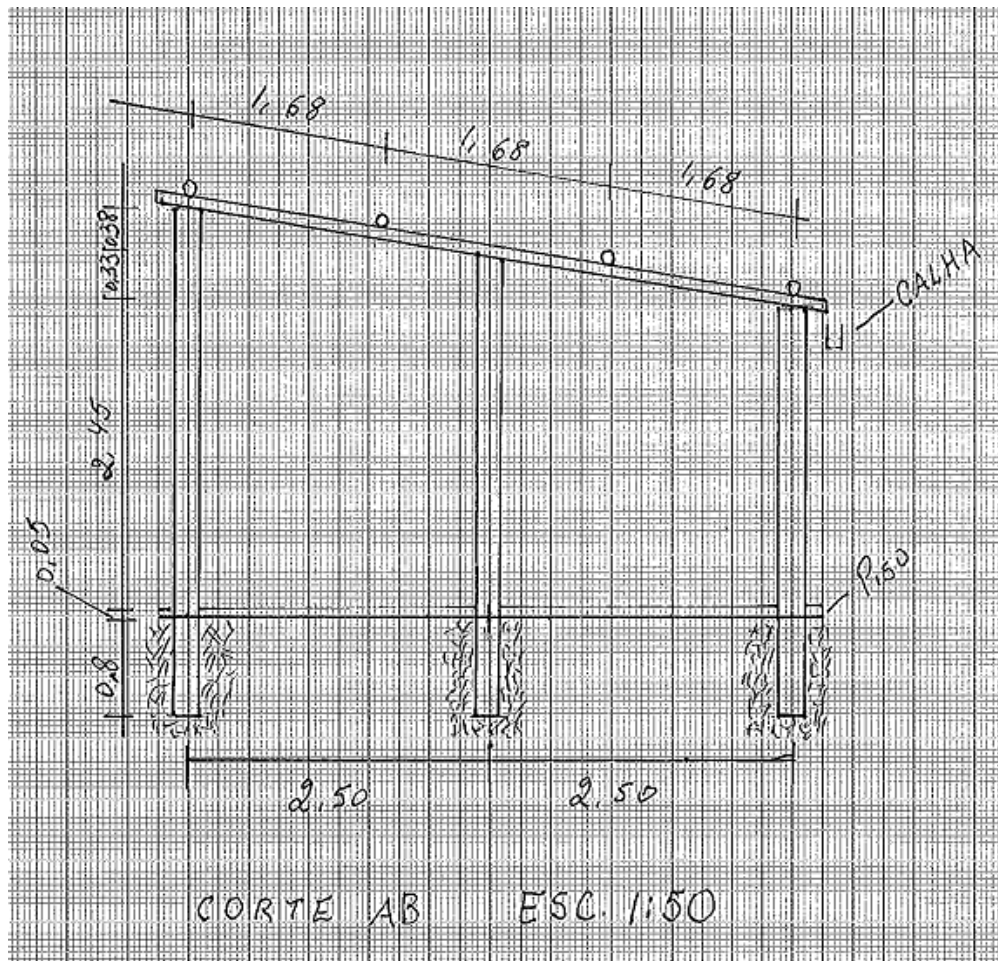
Figura 26 – Vista da estrutura de madeira em corte
