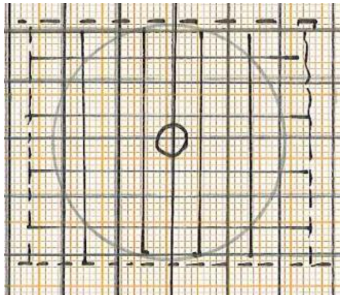
Figura 18 – Croquis da malha de ferro CA-60 5 mm para confecção da coroa. As varetas devem ser dispostas 10 cm umas das outras e amarradas com arame recozido.
